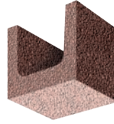
L x B x H in cm: 24,0 x 24,0/30,0/36,5 x 24,8 Betonquerschnitte: 9,5/17; 12,5/17; 18/17; 21/17
