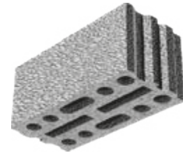
L x B x H in cm: 49,7 x 24,0 x 23,8 16 DF
