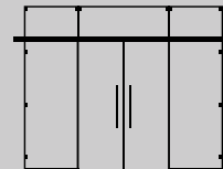
2-FLG. SCHIEBETÜR MIT ZWEI FESTEN SEITENTEILEN UND OBERLICHT 2-WING SLIDING DOOR WITH TOP LIGHT AND TWO FIXED SIDE SECTIONS
