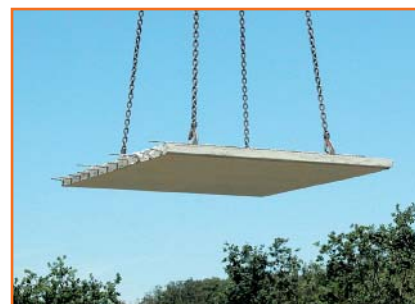
3. Auflegen der Deckenelemente auf die Montageunterstützung.
